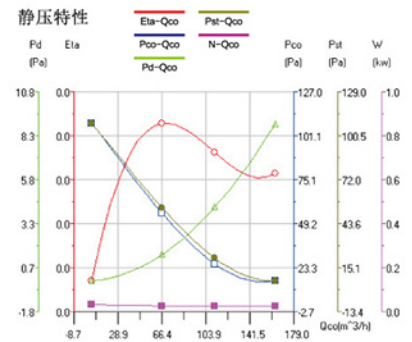
静压特性
