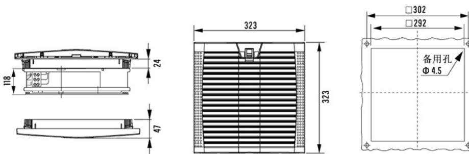
尺寸图
