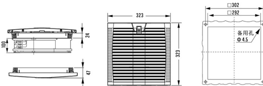
尺寸图
