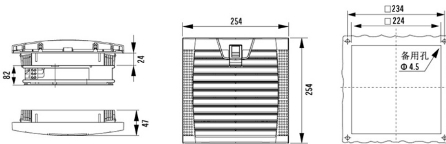
尺寸图
