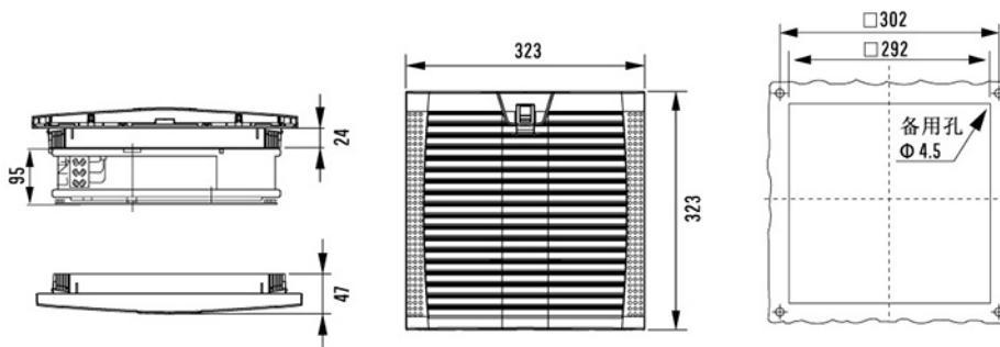
尺寸图
