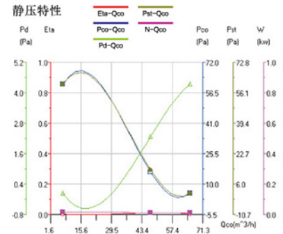
静压特性
