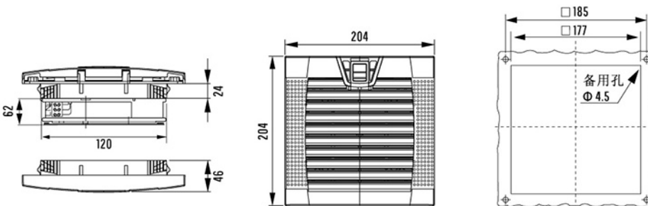
尺寸图
