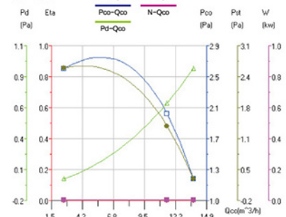
静压特性
