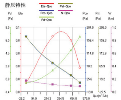
静压特性
