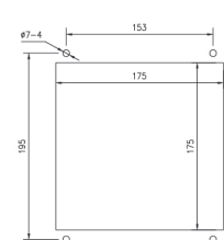
开孔尺寸
