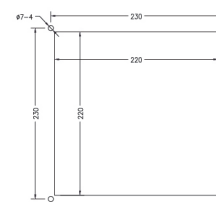
开孔尺寸
