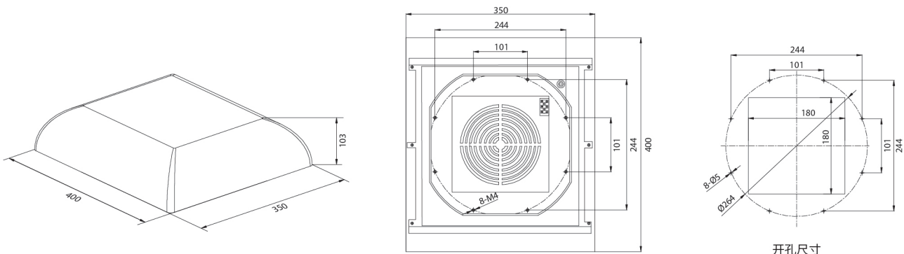
开孔尺寸
