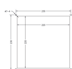
开孔尺寸
