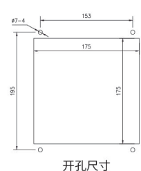
开孔尺寸
