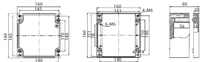
LK161609产品尺寸及安装孔位置
