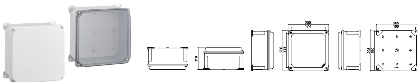
外形尺寸、安装孔及孔位图
