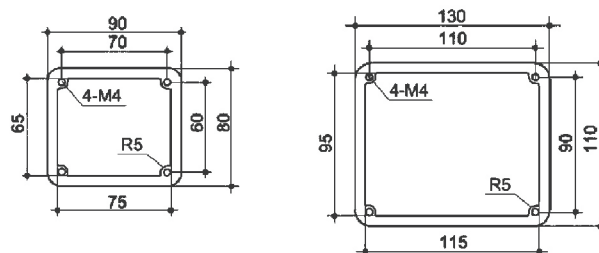
LK0908配电箱透明窗
