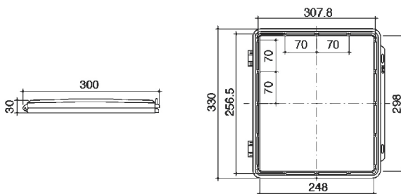
LK4-26B产品外形尺寸、安装孔位图
