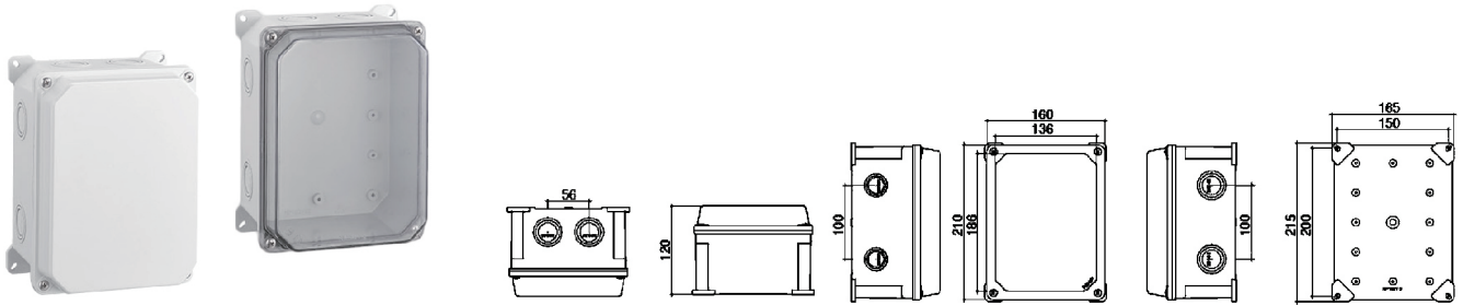
外形尺寸、安装孔及孔位图
