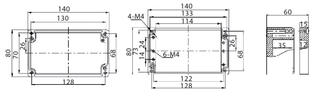
LK140806产品尺寸及安装孔位置
