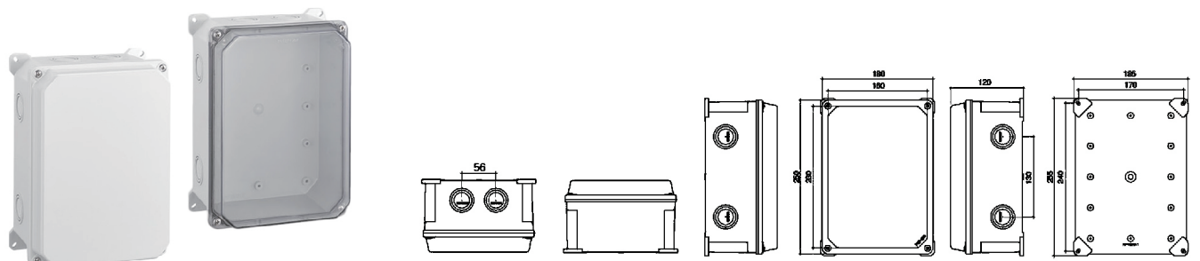
外形尺寸、安装孔及孔位图
