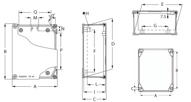
KPA11/12/13/14/15/16 尺寸、安装孔及安装孔位置
