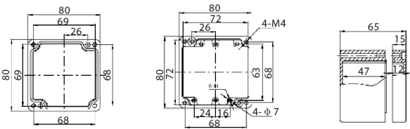
LK080807产品尺寸及安装孔位置
