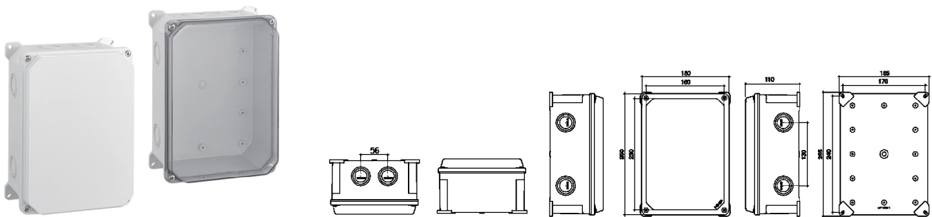
外形尺寸、安装孔及孔位图
