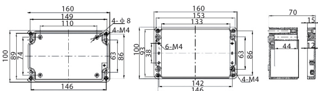
LK161007产品尺寸及安装孔位置
